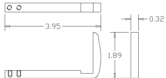
BOTTOM BLADE
